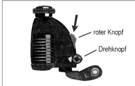
Der Seitendynamo wird durch Drücken auf den roten Knopf eingeschaltet. Zum Ausschalten wird er vom Rad weggeschwenkt.
